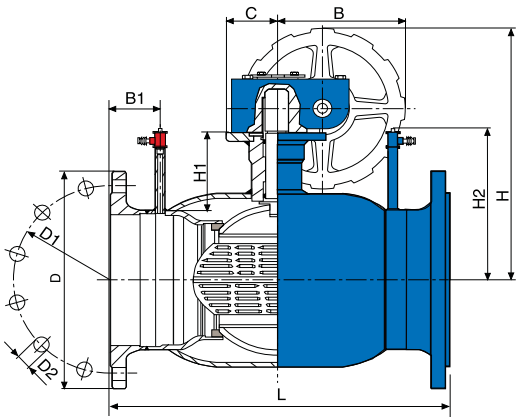
KOŁNIERZE WG: EN1092-1
