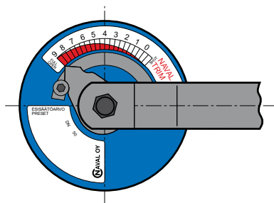
SKALA REGULACYJNA (Z RĄCZKĄ) DN40-250
