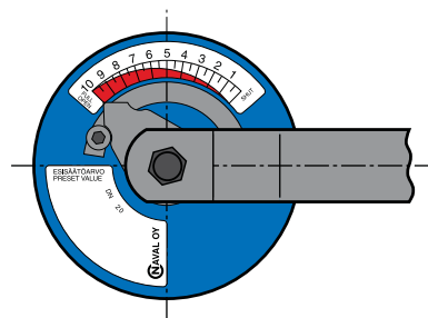
SKALA REGULACYJNA (Z RĄCZKĄ) DN15-32
