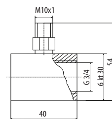
Trójnik DN20 do montażu czujnika temperatury w osłonie
