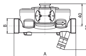
Widok przetwornika z boku
