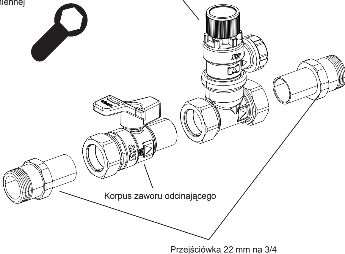
Klucz montażowy 4807.00.906 główicy wymiennej
