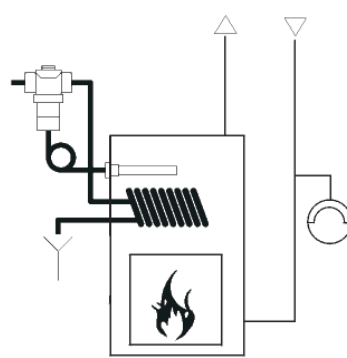
rys.3 Instalacja z naczyniem wzbiorczym systemu otwartego
