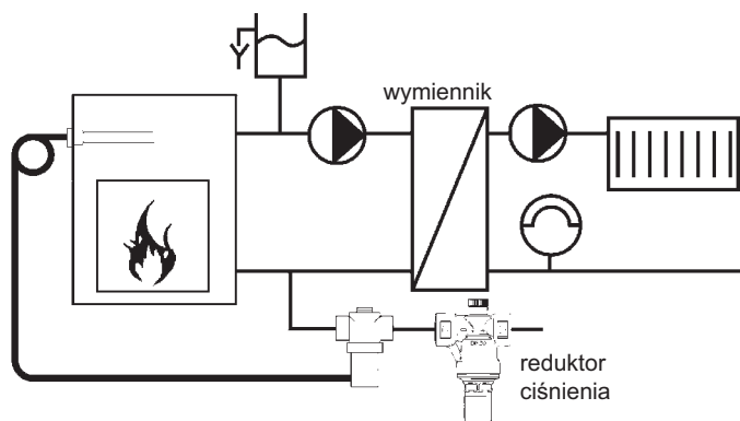
rys.3 Instalacja z naczyniem wzbiorczym systemu otwartego
